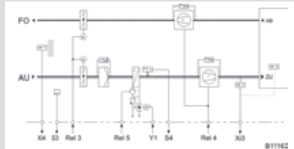
Regulación constante de la temperatura del aire (salas)
