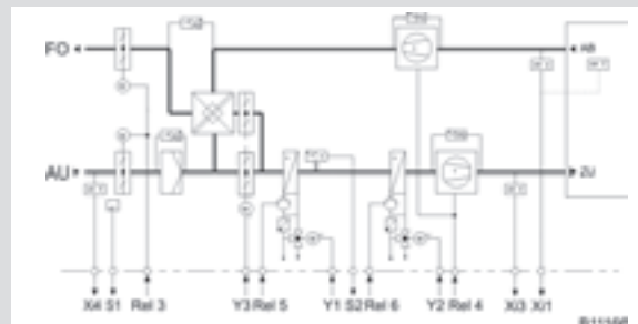
Regulación en cascada del control de la extracción/suministro de aire para calefacción/climatización con recuperación de calor
