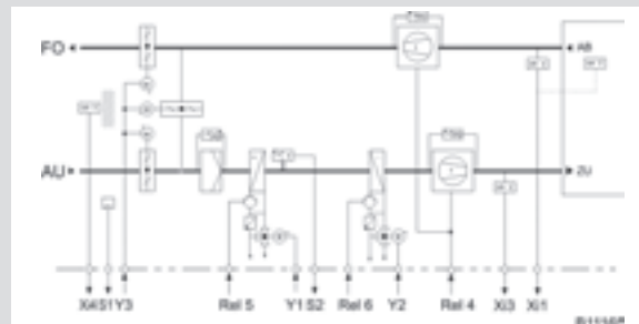
Regulación en cascada del control de la extracción/suministro de aire (salas), con función de circulación de aire
