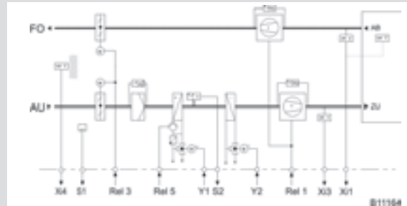
Regulación en cascada del control de la extracción/suministro de aire (salas) para calefacción/climatización
